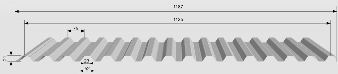
Chevauchement d'une nervure
