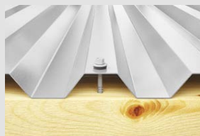
Fissaggio su legno
